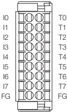
FX5-SF-8DI4
