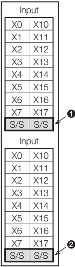
FX5-C32EX/DS-TS
