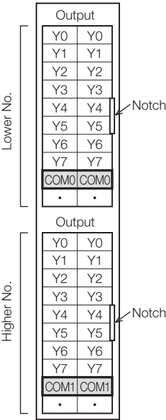
FX5-C32EYT/D
