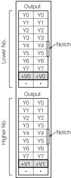
FX5-C32EYT/DSS
