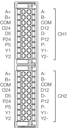
FX5-2HC/ES
