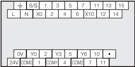
FX5UJ-24MT/ESS
