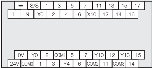
FX5S-30MT/ESS
