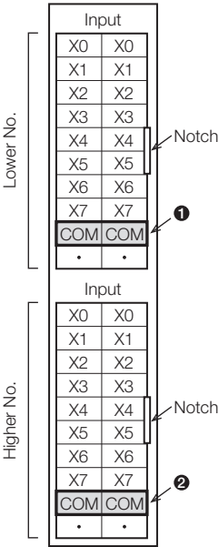
FX5-C32EX/D
