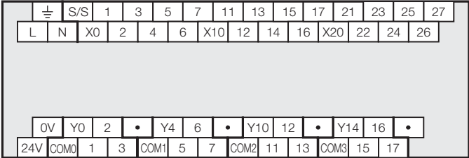
FX5UJ-40MT/ESS
