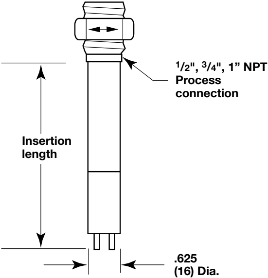
Mini Sensor (TXM)
