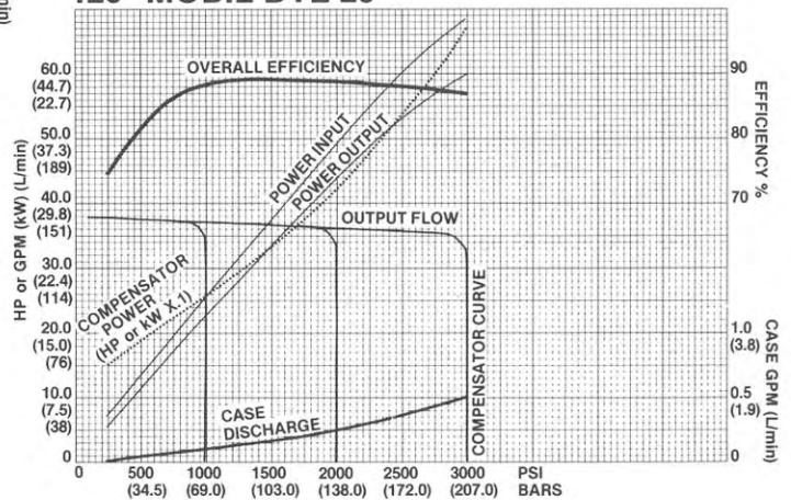
PV 420 2200 RPM 120° MOBIL DTE 26
