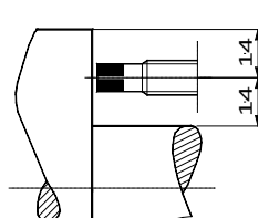
Abstand zur Wellenschulter Sensor parallel zu elektrisch leitfähigem Material Distance to shaft shoulder Sensor parallel to electrically conducting material Distance à l'épaule d'arbre Capteur monté en parallèle à un matériel conductif
